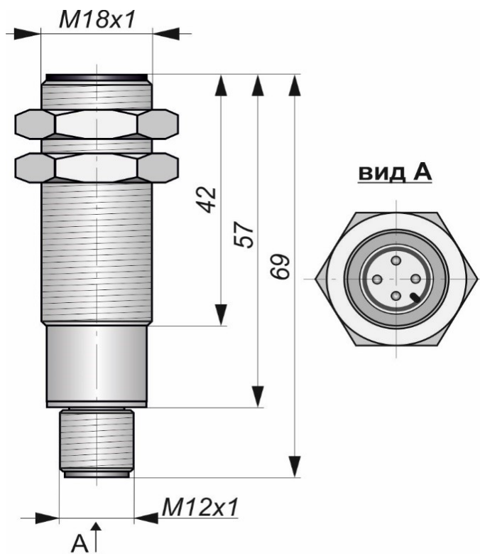
Габаритный чертеж
