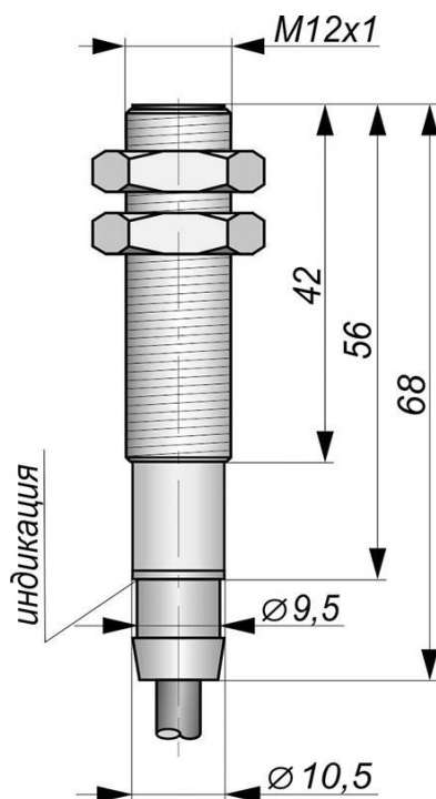
Габаритный чертеж
