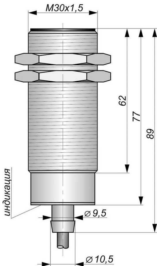
Габаритный чертеж
