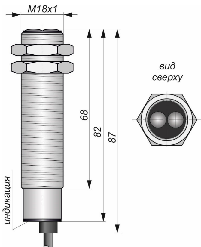
Габаритный чертеж
