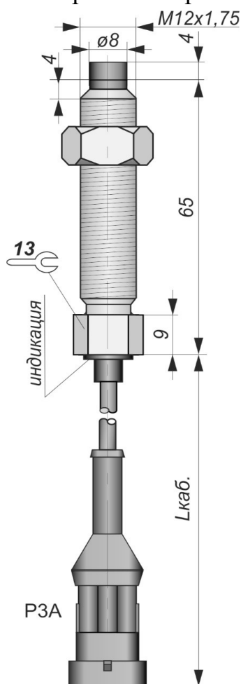
Габаритный чертеж
