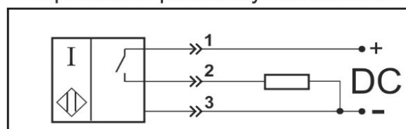
Нормально-разомкнутый контакт
