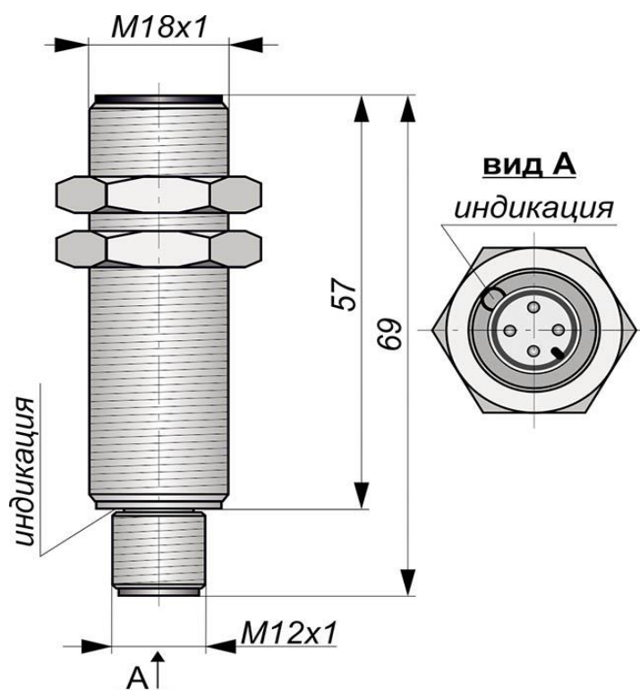
Габаритный чертеж
