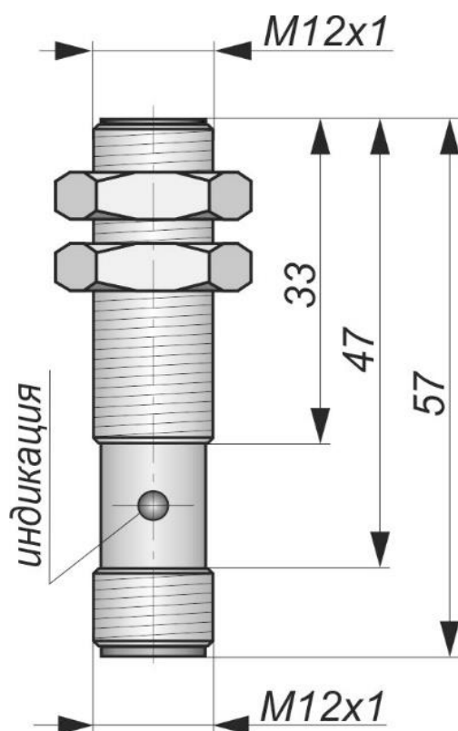
Габаритный чертеж
