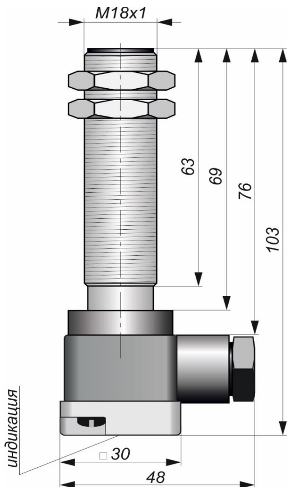
Габаритный чертеж
