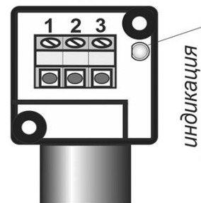
Цоколевка клеммной колодки
