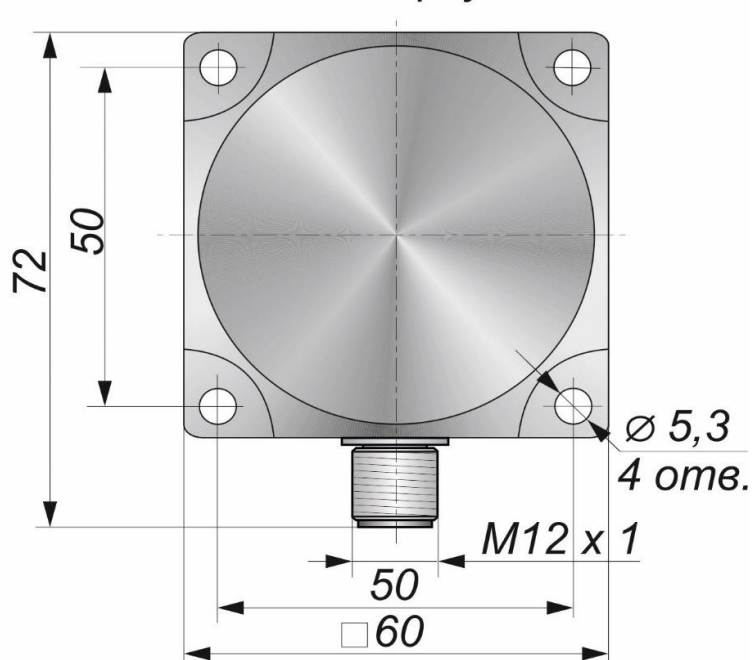
Габаритный чертеж
