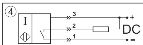
Нормально-разомкнутый контакт
