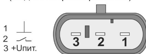
Нормально-разомкнутый контакт
