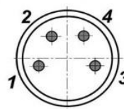
Цоколевка разъема
