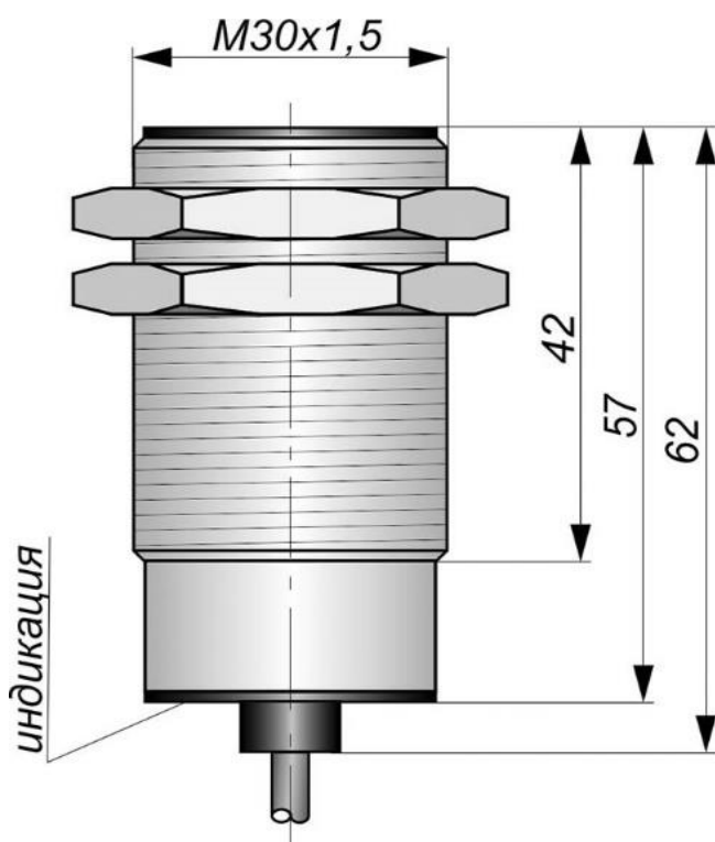
Габаритный чертеж
