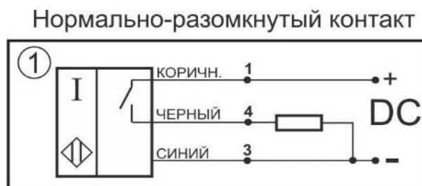
Схема соединения
