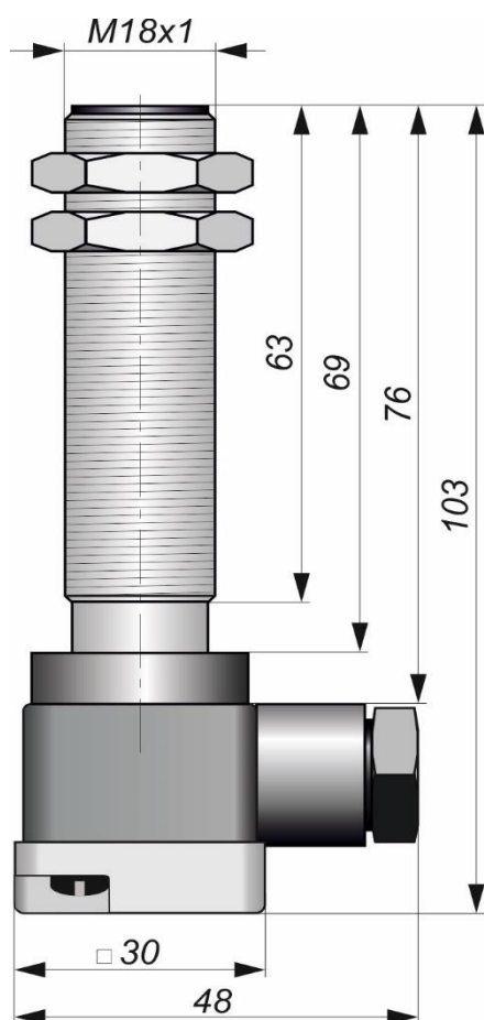
Габаритный чертеж
