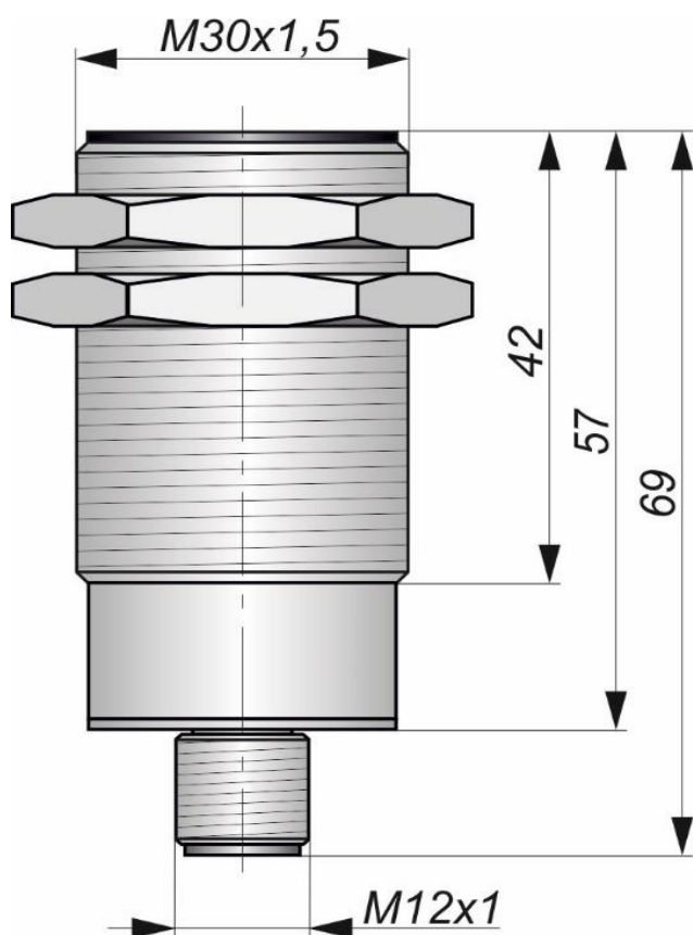
Габаритный чертеж
