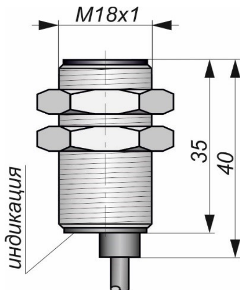
Габаритный чертеж
