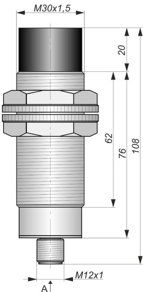
Габаритный чертеж
