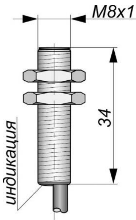
Габаритный чертеж
