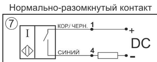
Схема соединения
