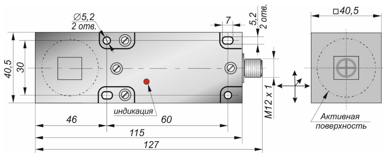
Габаритный чертеж
