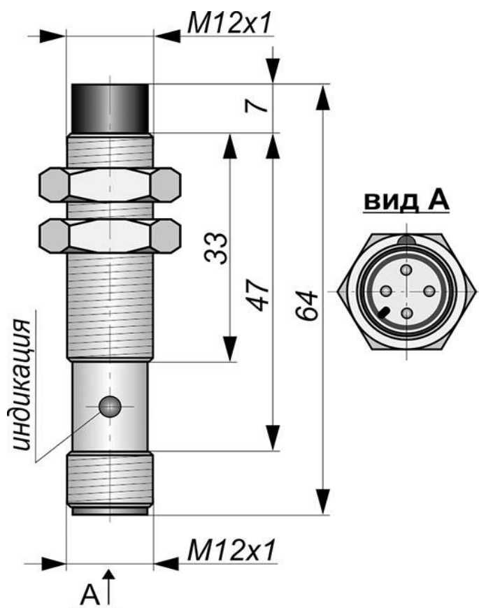
Габаритный чертеж
