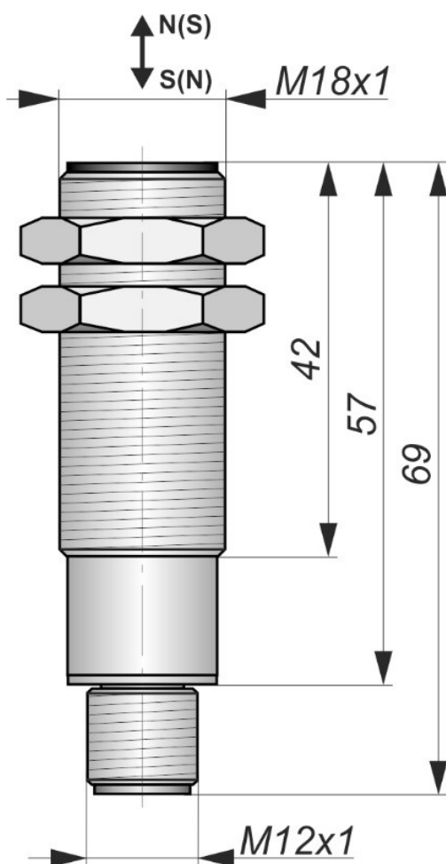
Габаритный чертеж
