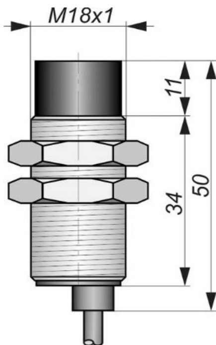
Габаритный чертеж
