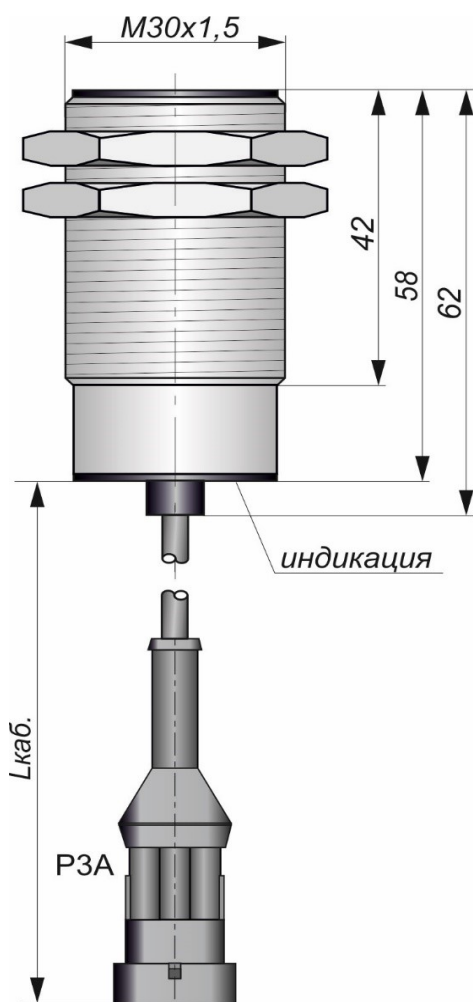
Габаритный чертеж
