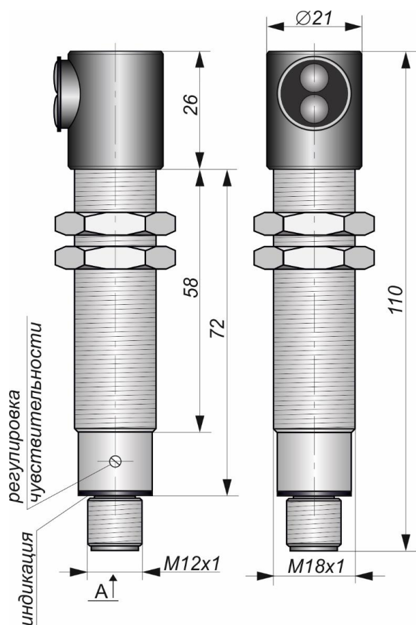
Габаритный чертеж
