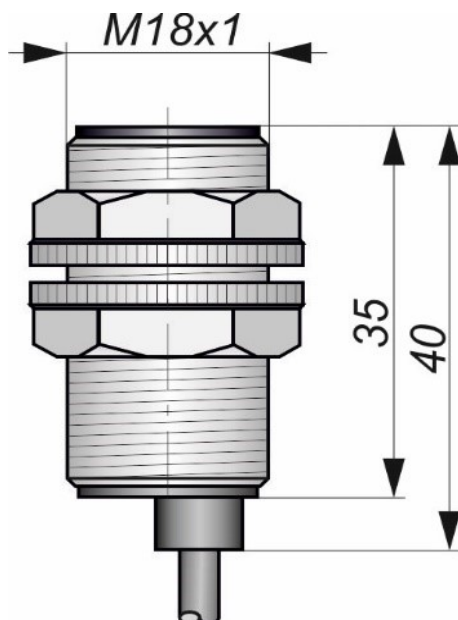
Габаритный чертеж
