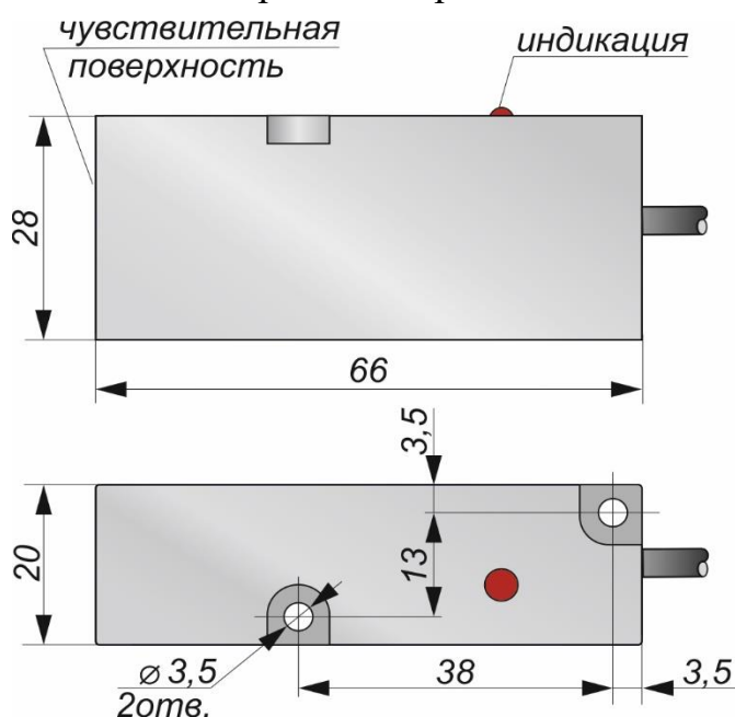
Габаритный чертеж
