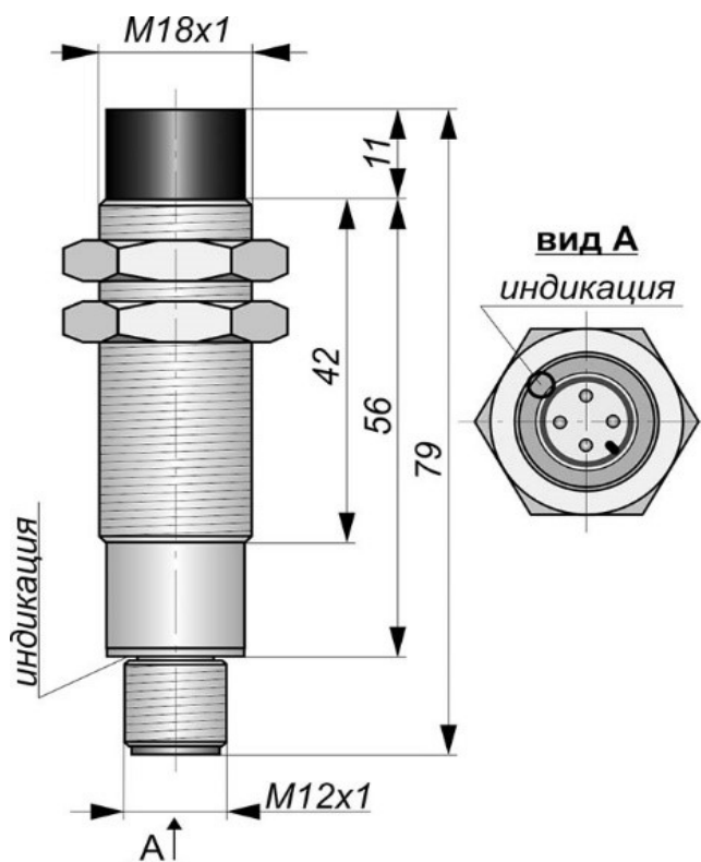
Габаритный чертеж
