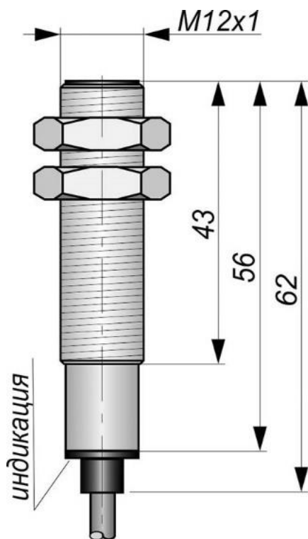
Габаритный чертеж
