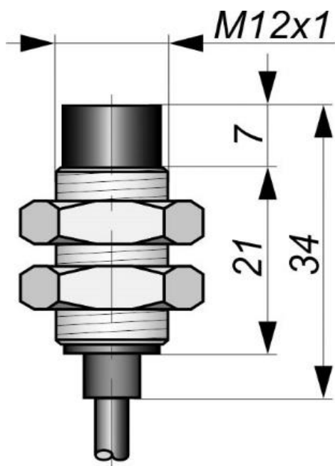
Габаритный чертеж
