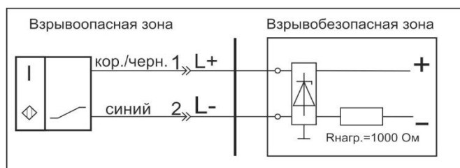
Схема соединения
