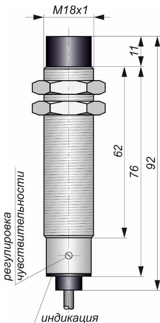
Габаритный чертеж
