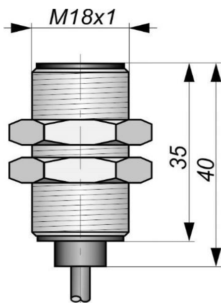
Габаритный чертеж
