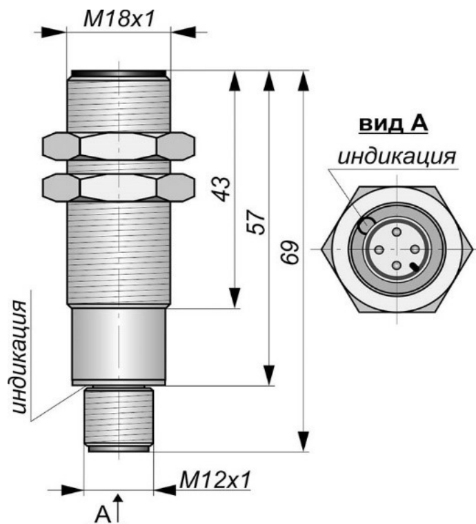
Габаритный чертеж
