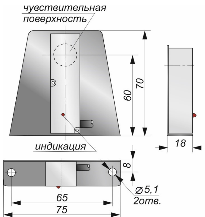
Габаритный чертеж
