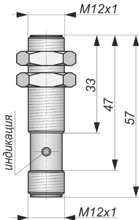
Габаритный чертеж
