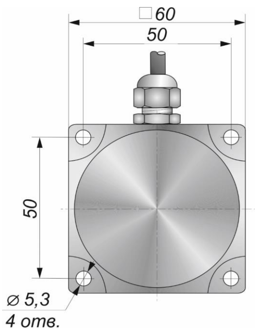
Габаритный чертеж
