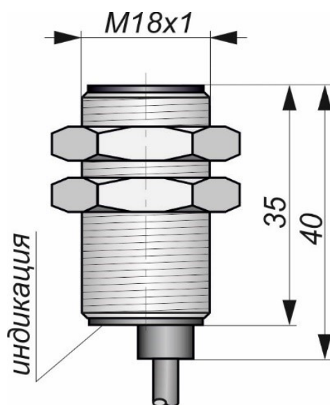
Габаритный чертеж
