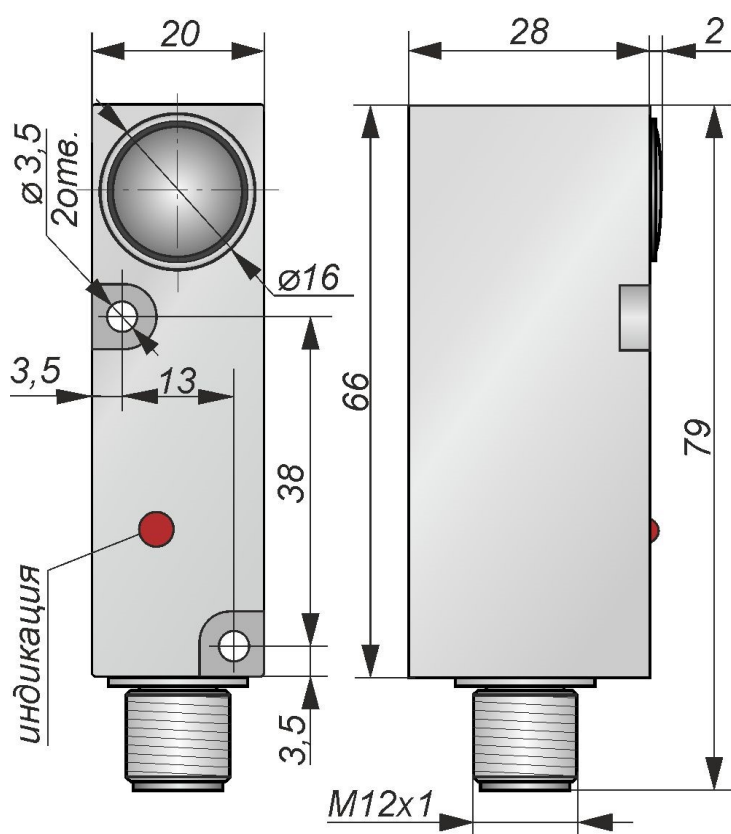
Габаритный чертеж
