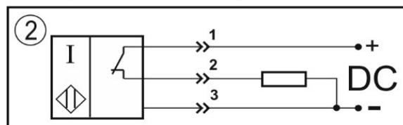
Цоколевка разъема
