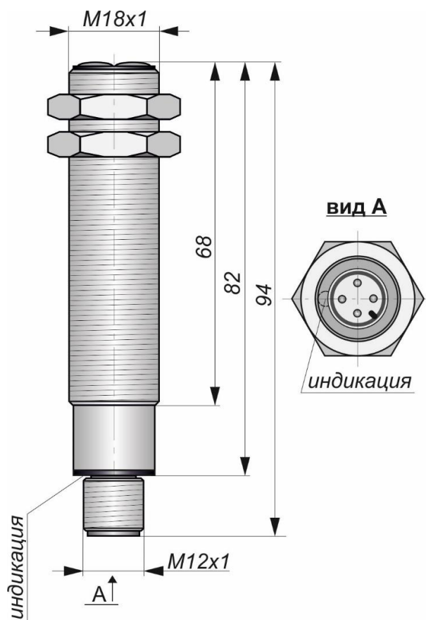
Габаритный чертеж
