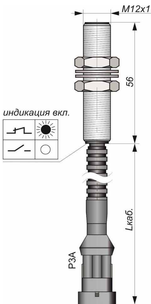
Габаритный чертеж
