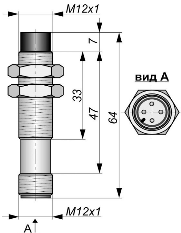
Габаритный чертеж
