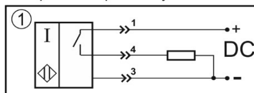
Цоколевка разъема
