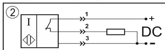
Нормально-замкнутый контакт
