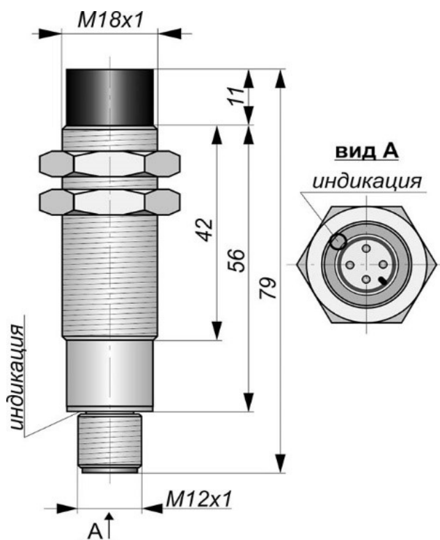
Габаритный чертеж
