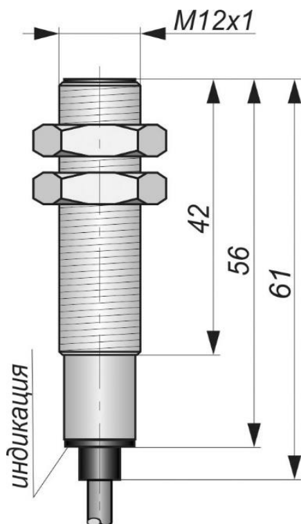
Габаритный чертеж
