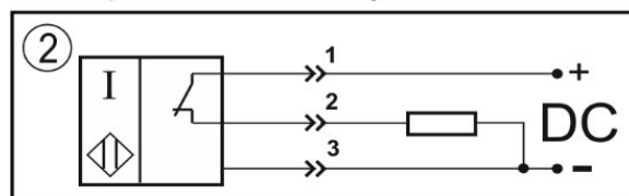
Нормально-замкнутый контакт
