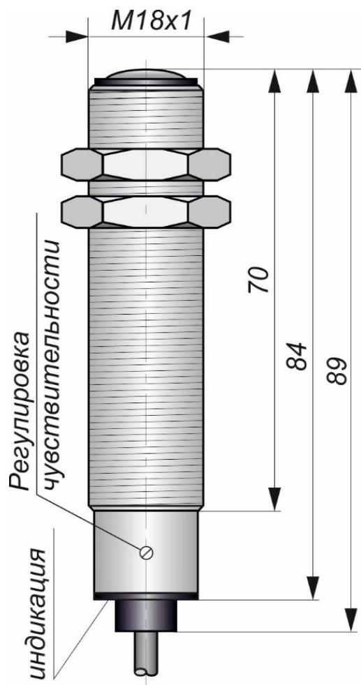
Габаритный чертеж
