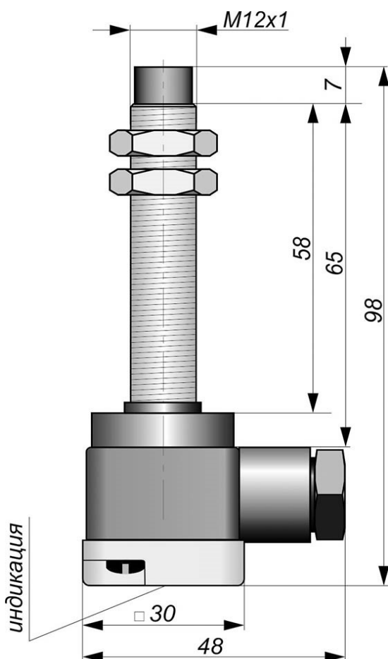
Габаритный чертеж
