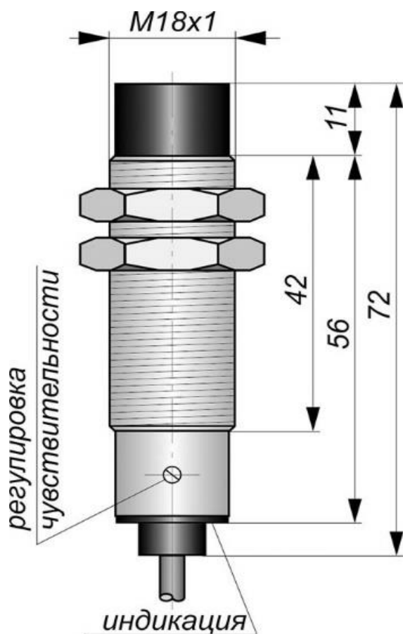
Габаритный чертеж
