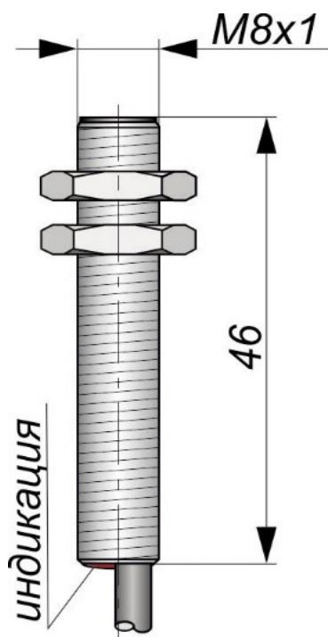
Габаритный чертеж
