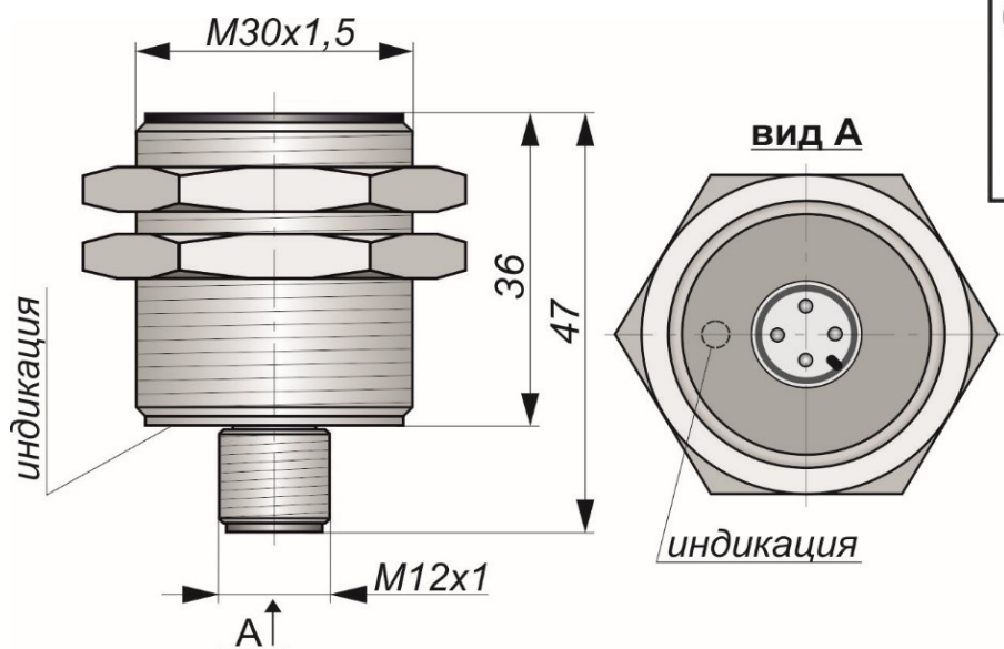
Габаритный чертеж
